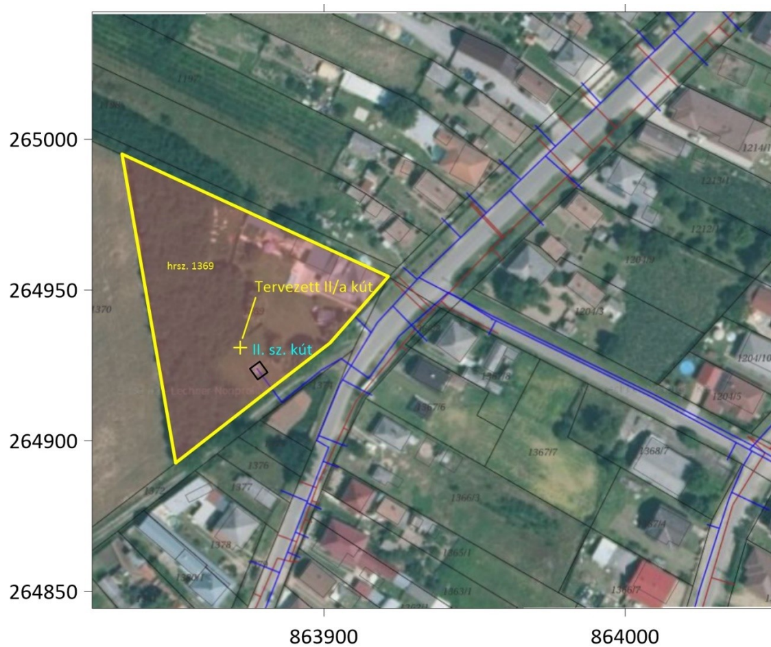
A II.sz. kút (B-31) melléfúrásos felújításának javasolt helye.
