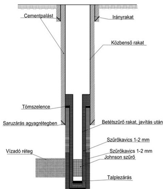
Betétészűrő cserével javított kútszerkezet
