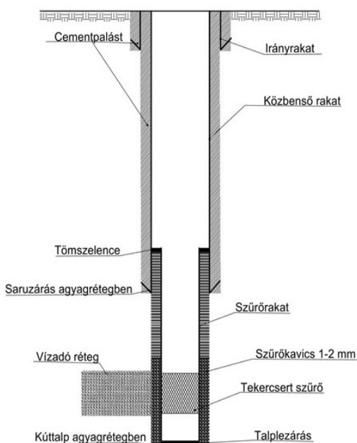
Melléfúrásos felújítás kútszerkezete
